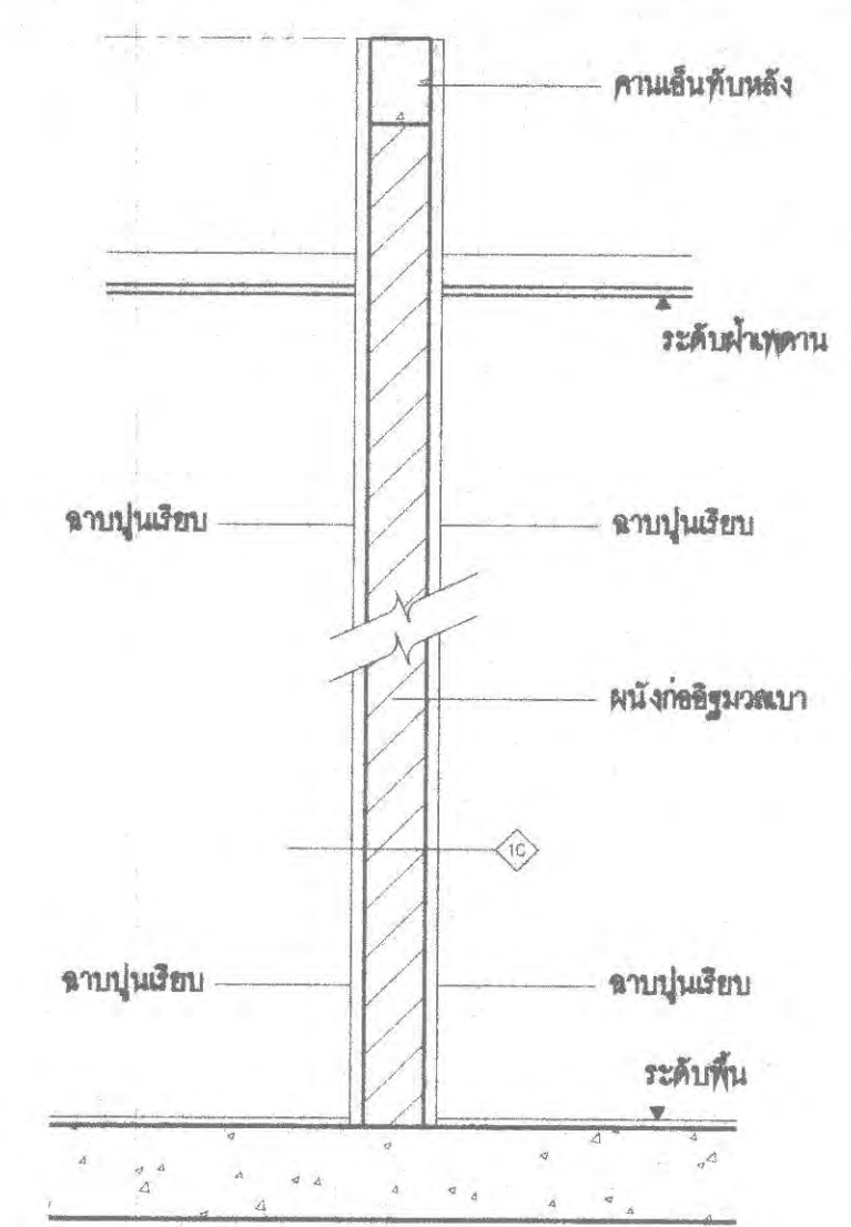
1 ผนังก่ออิฐฉาบปูนหนา 12.5 CM ฉาบปูน 2 ด้าน สูงกว่าระดับฝ้าเพดาน 300 มม
