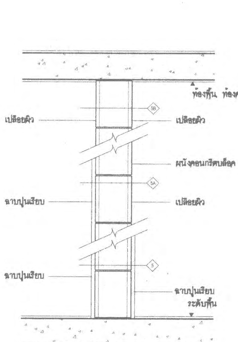
ผนังแบบที่ 5 ผนังฉาบปูนเสริมเหล็กหนา 8"
