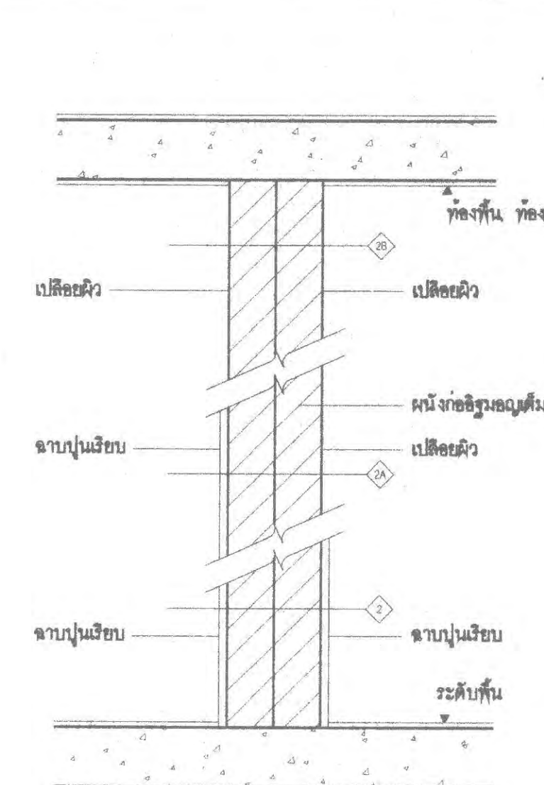
ผนังแบบที่ 2 ผนังฉาบปูนเต็มแผ่น
