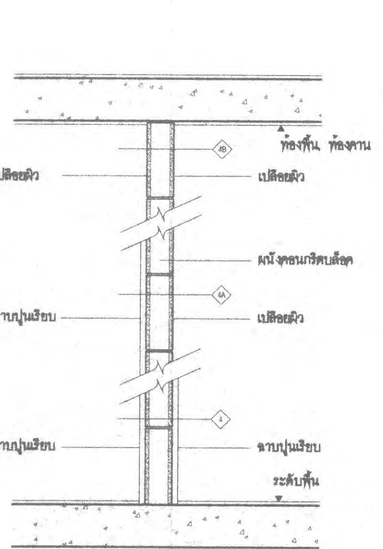
ผนังแบบที่ 4 ผนังฉาบปูนเสริมเหล็กหนา 3"
