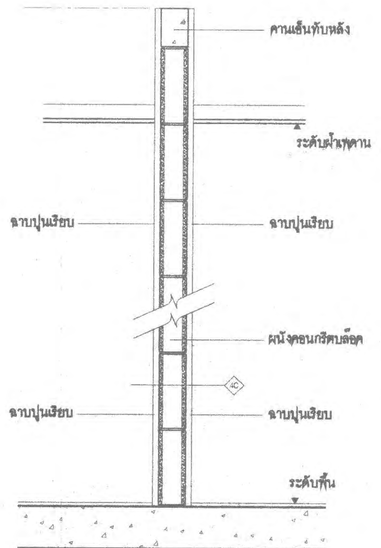
1 ผนังฉาบปูนเสริมเหล็กหนา 3" ฉาบปูนเสริม 2 ด้าน สูงกว่าระดับฝ้าเพดาน 300 มม
