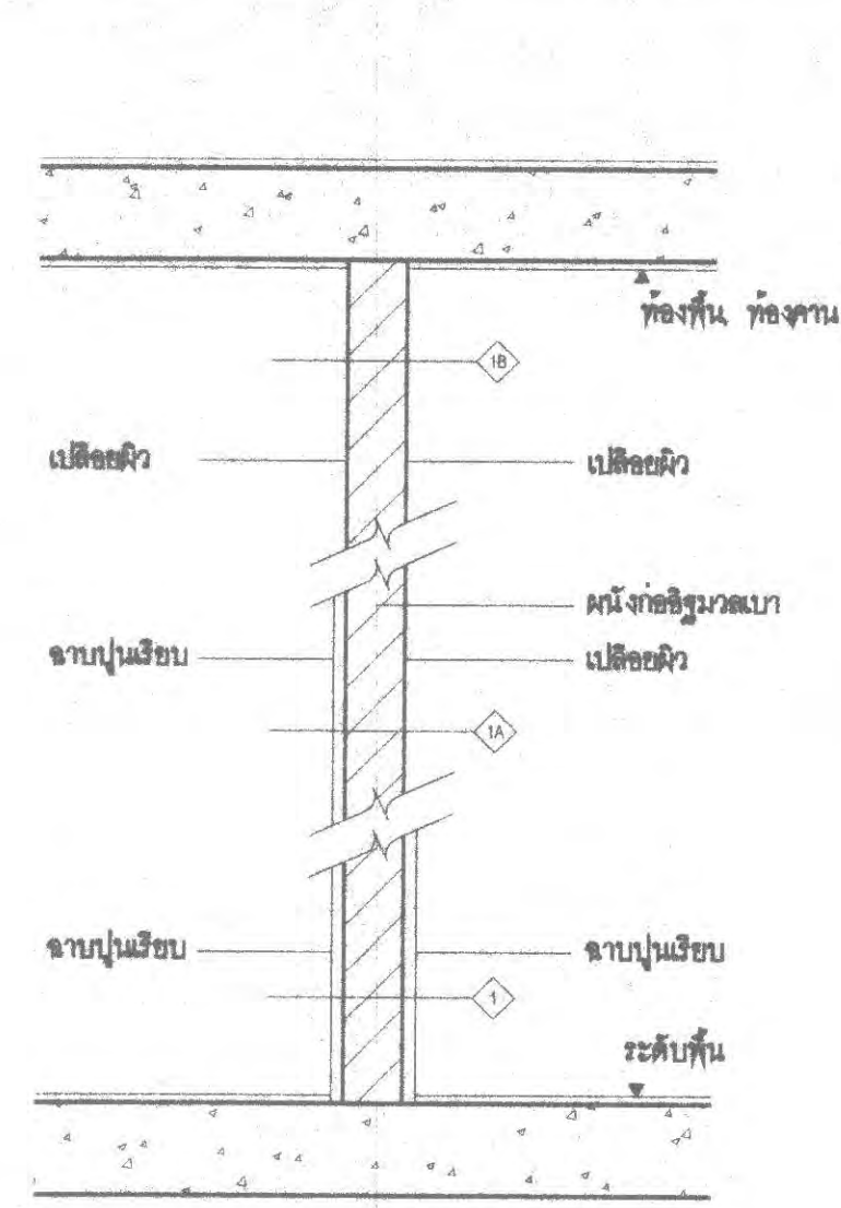
ผนังแบบที่ 1 ผนังก่ออิฐฉาบปูนหนา 12.5 CM
