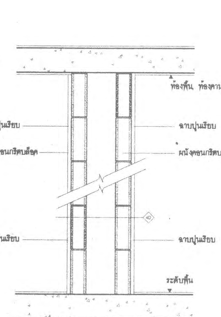
1 ผนังฉาบปูนเสริมเหล็กหนา 3" 2 ชั้น เติมน้ำหนัก ฉาบปูนเสริม 2 ด้าน
