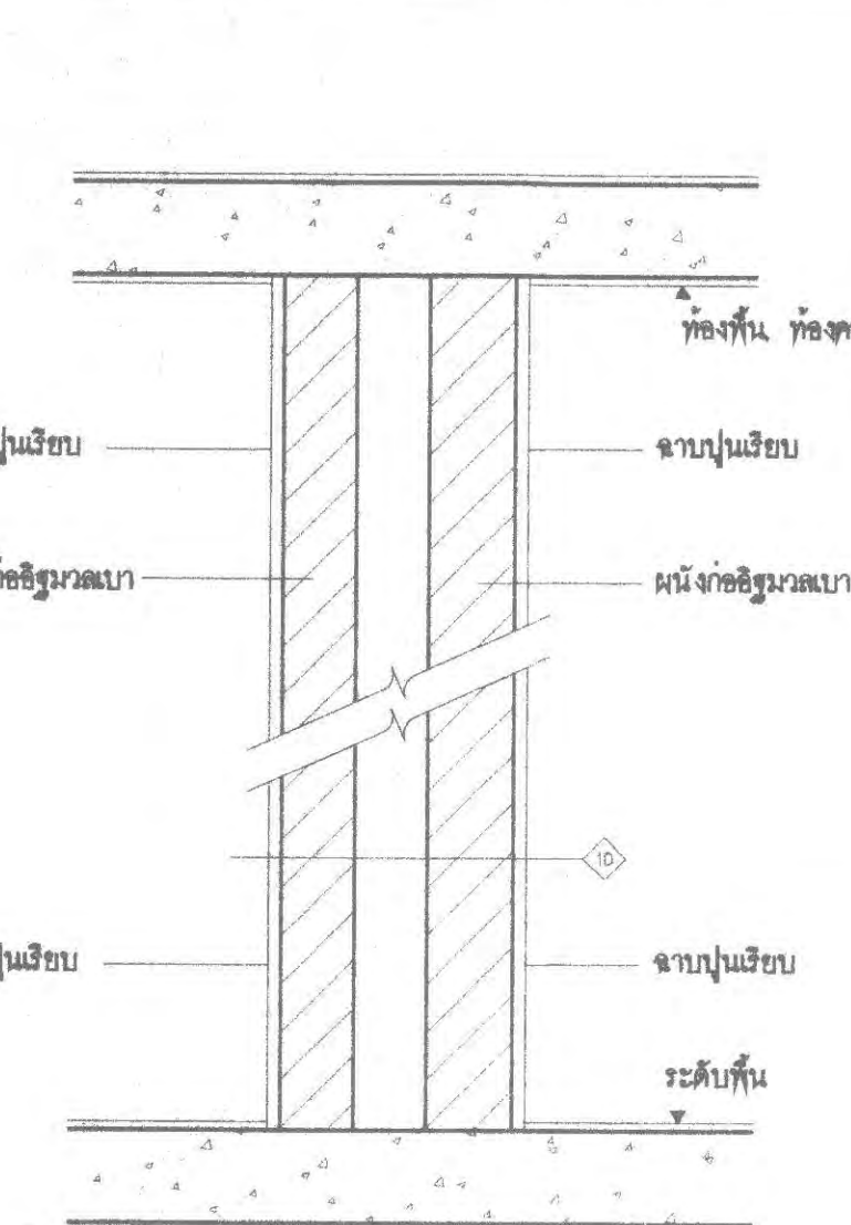
1 ผนังก่ออิฐฉาบปูนหนา 7.5 CM 2 ชั้น เติมน้ำหนัก ฉาบปูน 2 ด้าน
